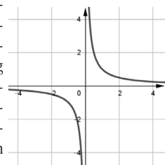
Figur 2. Grafen för en rationell funktion.
