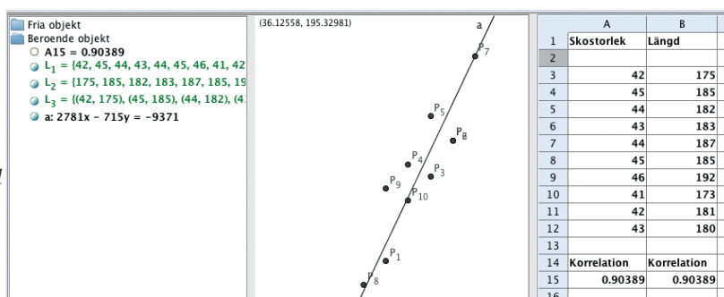
Figur 6: Korrelationen mellan längd och skorstorlek beräknad i GeoGebra samt regressionslinje genom punktmängden, med r = 0,90389 .
